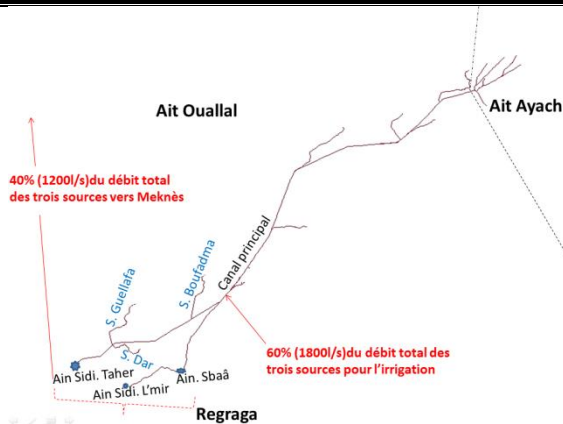
Figure5: Adduction de la ville Meknès en eau potable
